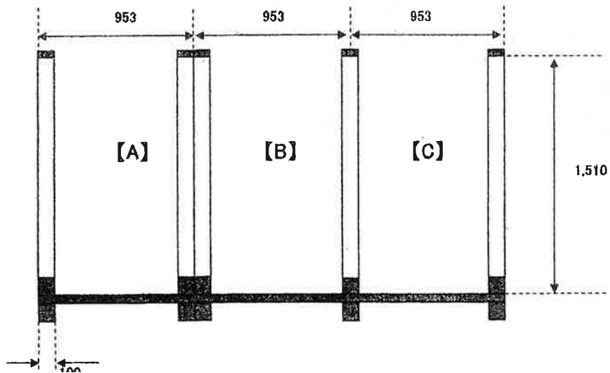
【正面】
