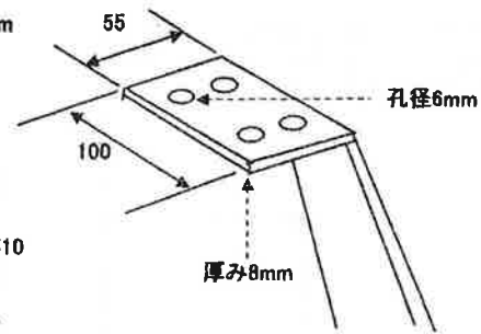
【下部取付】
