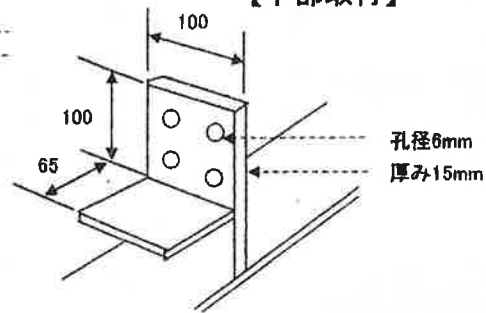
【下部取付】
